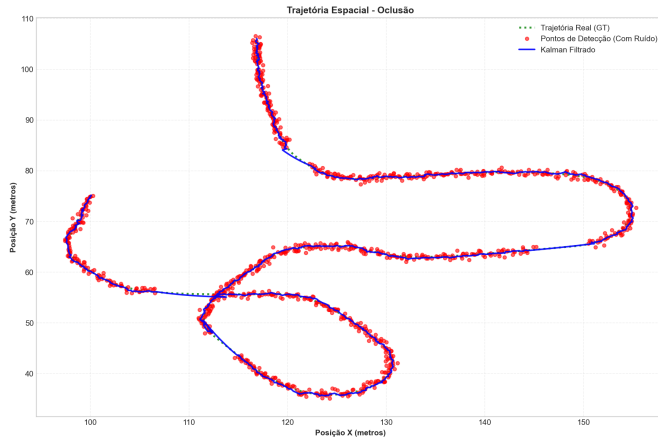
Figura 9: Estimativa espacial durante o Cenário 6. Nas zonas de oclusão (ausência de dados dos sensores), a estimativa PVA mantém a inércia da trajetória projetada em malha aberta.
