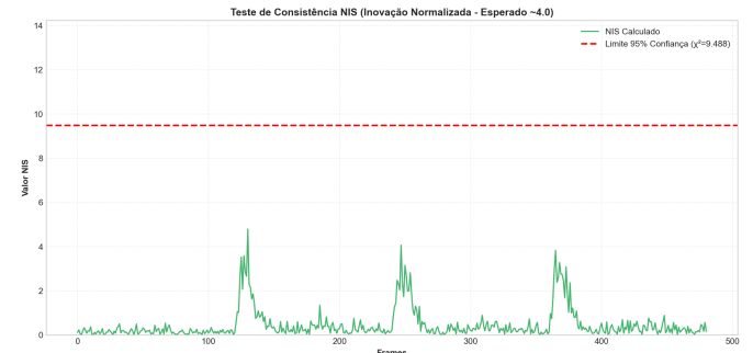
Figura 8: Histórico da métrica Normalized Innovation Squared (NIS) para o Cenário 2 Sintonizado. A linha pontilhada indica o limite estatístico de 9,49 (confiança de 95%).
